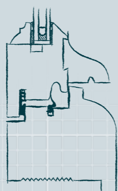
Traverse basse Pièce d'appui profilée. Possibilité de reproduction de l'existant.
