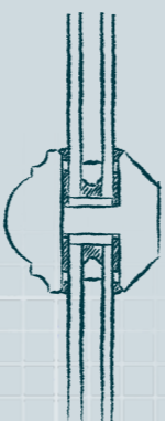
Petits bois Largeur 38 mm. Mortaisés. Assemblage à coupe d'onglet.
